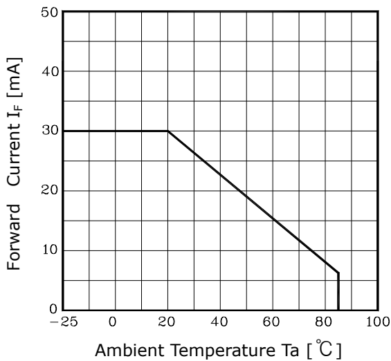
Fig. 3 I_F - T_a
