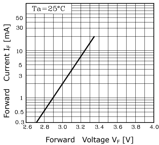
Fig. 1 I_F - V_F
