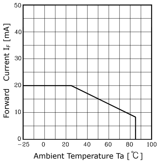
Fig. 3 I_F - T_a
