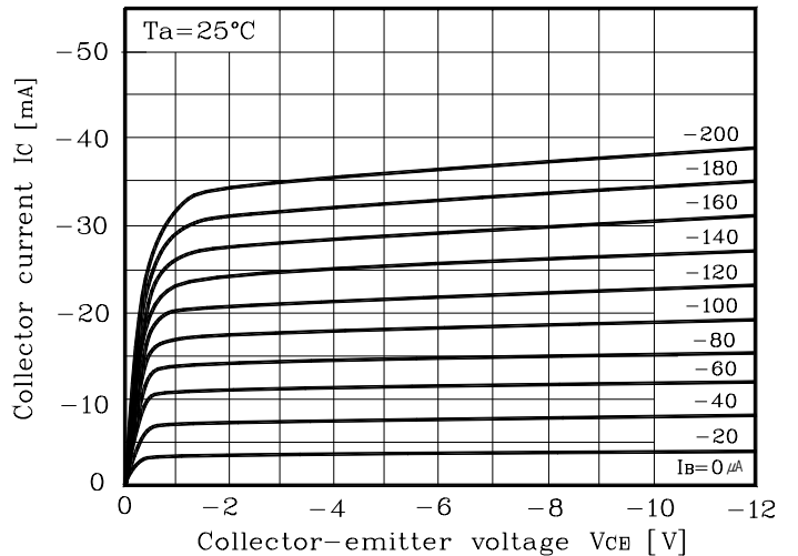
Fig. 2 I_C - V_{CE}
