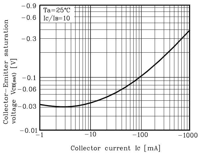
Fig. 3 V_{CE(sat)} - I_C
