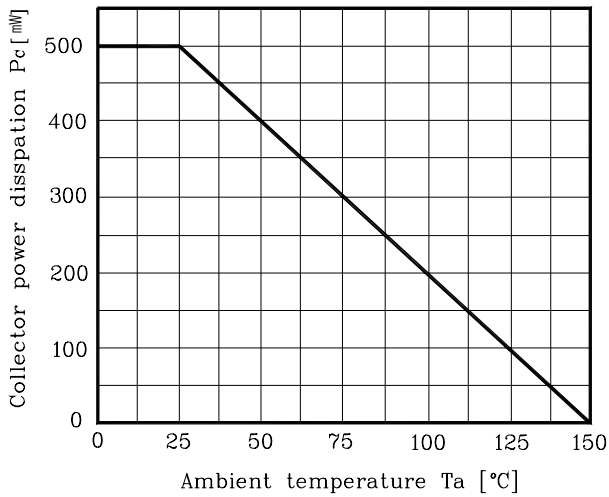
Fig. 1 P_C - T_a
