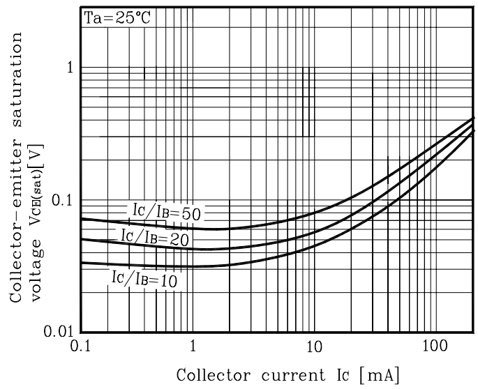
Fig. 4 V_{CE(sat)}-I_C
