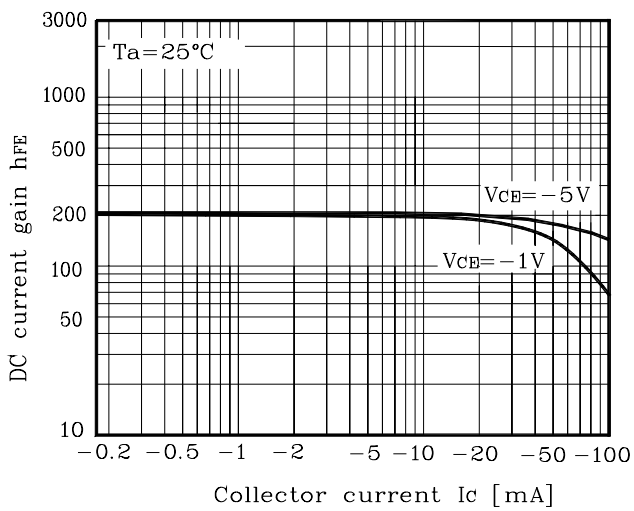
Fig. 3 h_{FE} - I_C
