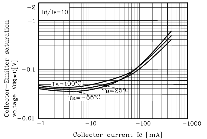
Fig. 4 V_{CE(sat)} - I_C
