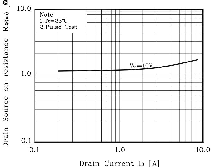
Fig. 3 R_{DS(on)} - I_D
