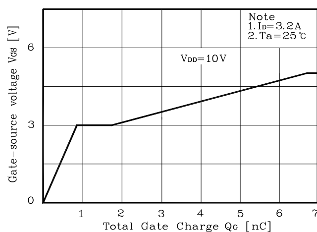
Fig. 6 V_{GS} - Q_G
