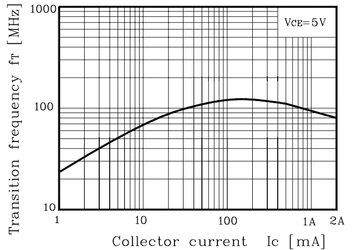
Fig. 4 f_T - I_C
