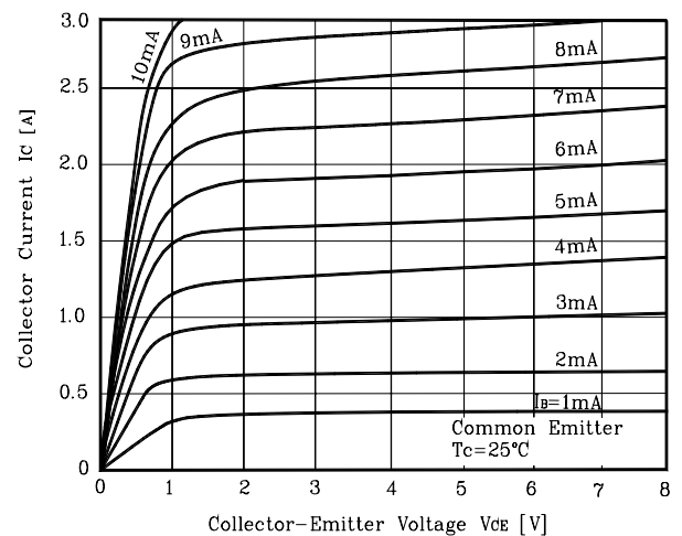
Fig. 4 I_C - V_{CE}
