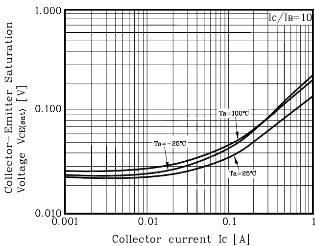
Fig. 5 I_C - V_{CE}
