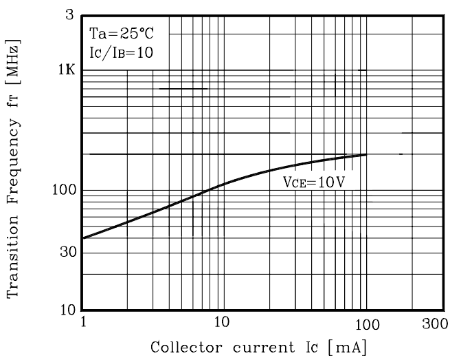
Fig. 9 f_T - I_C
