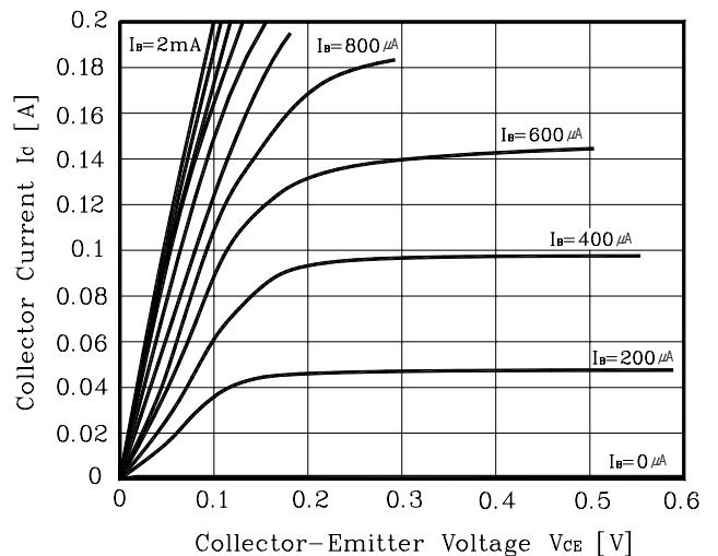
Fig. 6 I_C - V_{CE}
