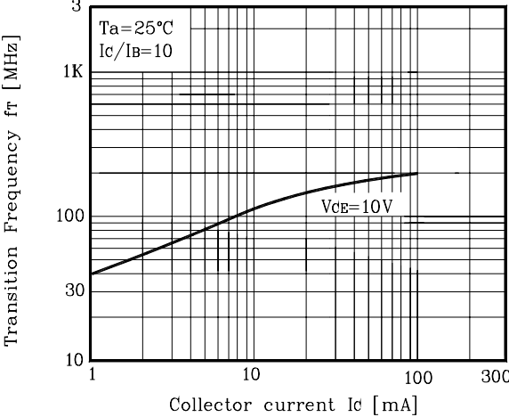
Fig. 7 f_T - I_C
