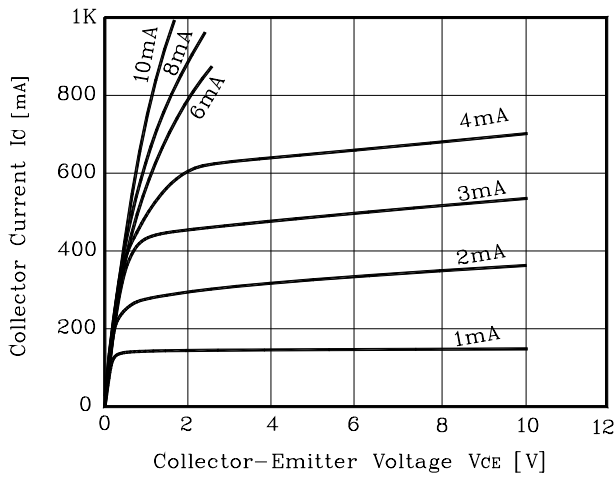
Fig. 5 I_C - V_{CE}
