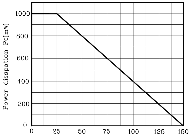
Fig. 1 P_C - T_a
