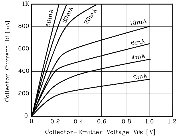
Fig. 6 I_C - V_{CE}
