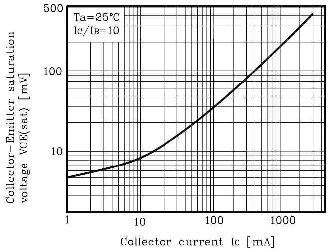
Fig. 1 V_{CE(sat)} - I_C
