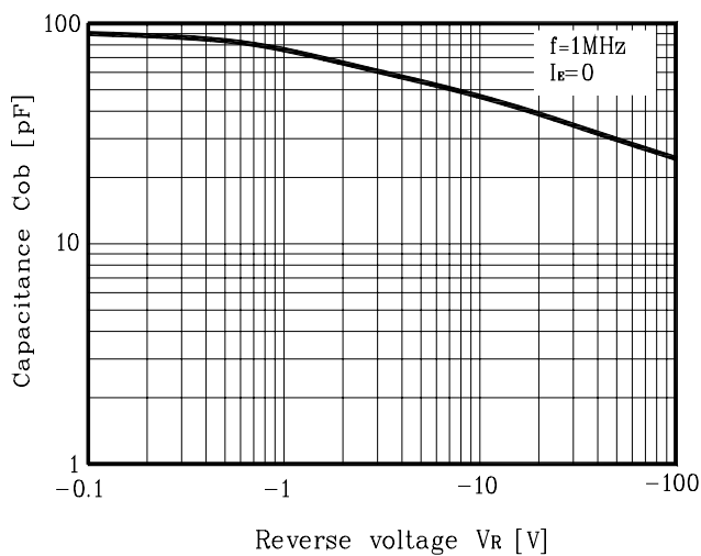
Fig. 5 C_{ob} - V_R
