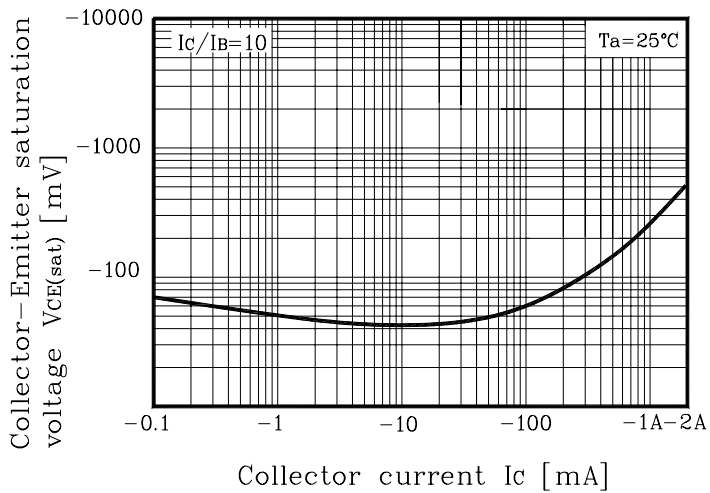
Fig.3 V_{CE(sat)} - I_C
