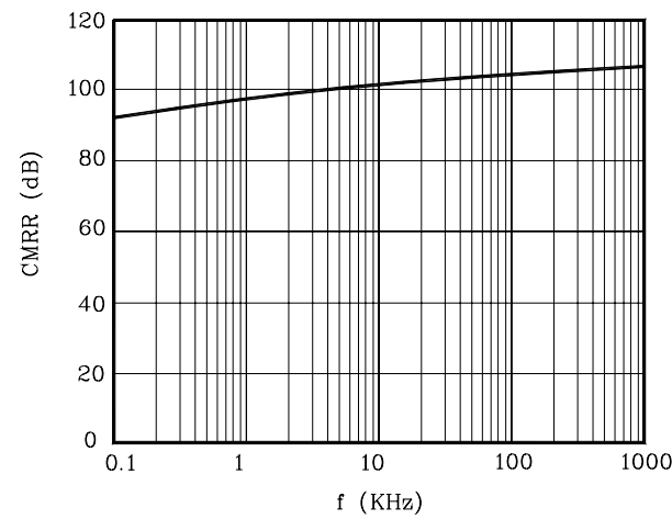
Fig. 5 CMRR-f
