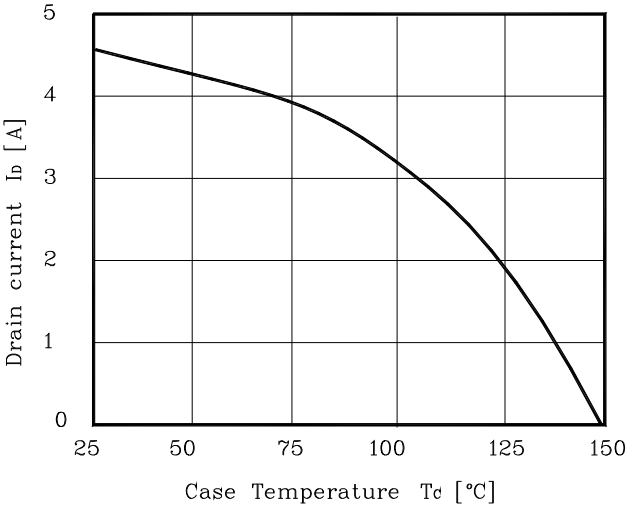
Fig. 9 I_D - T_C
