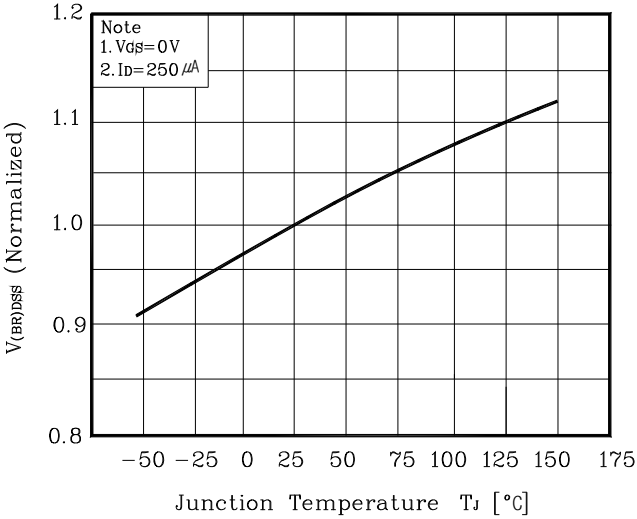
Fig. 7 V_{(BR)DSS} - T_J
