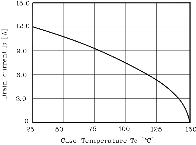
Fig. 9 I_D - T_C
