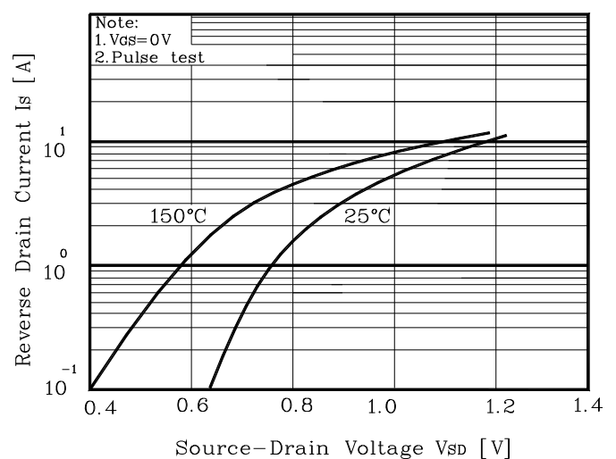
Fig. 4 I_S - V_{SD}
