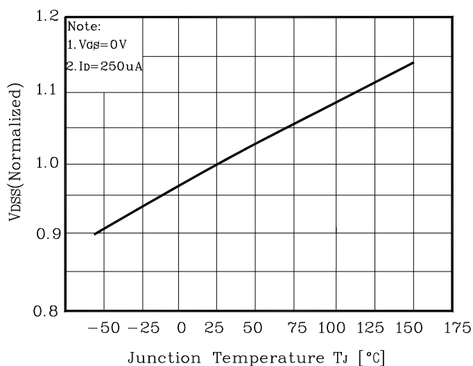
Fig. 7 V_{DSS} - T_J
