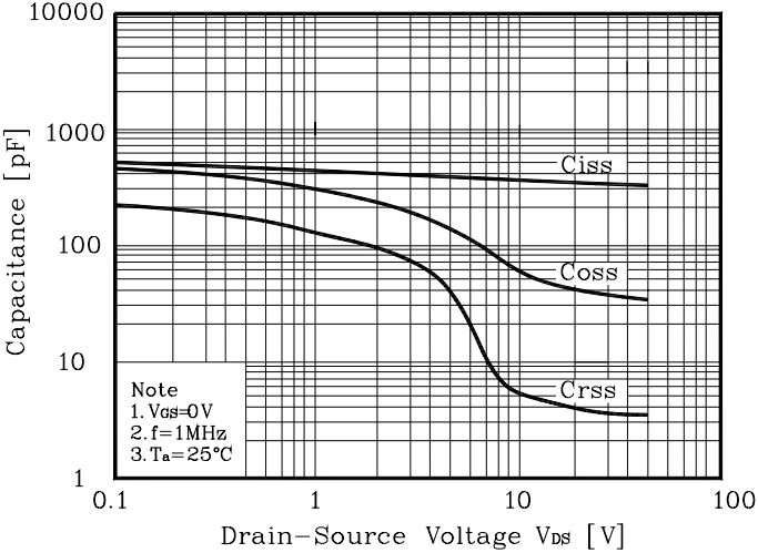
Fig. 5 Capacitance - V_{DS}
