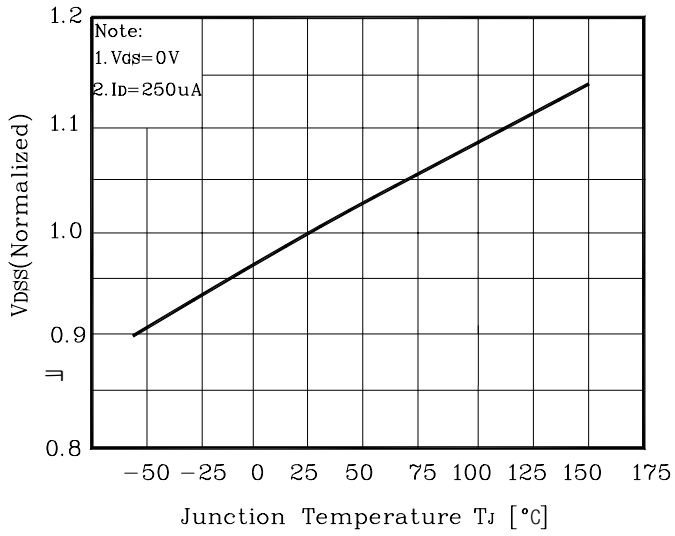
Fig. 7 V_{DSS} - T_J
