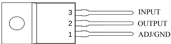
PKG : TO-220F-3L
