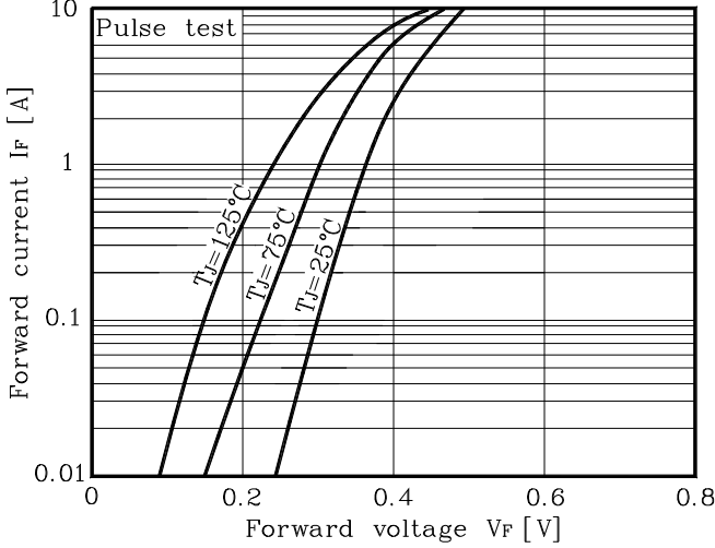
Fig. 1 I_F - V_F
