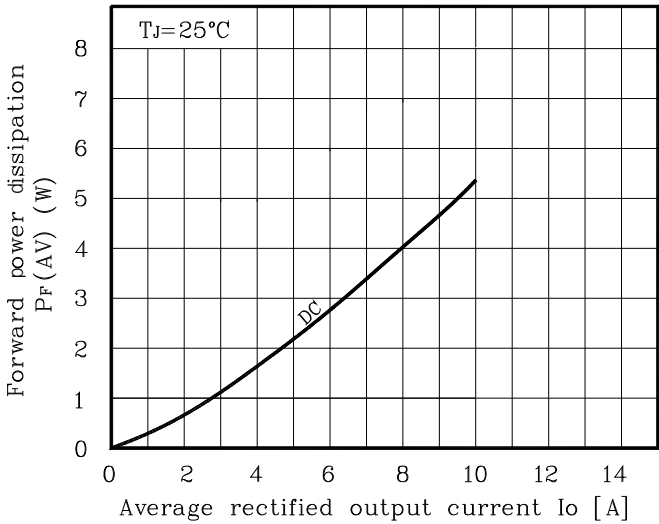
Fig. 3 P_F - I_O
