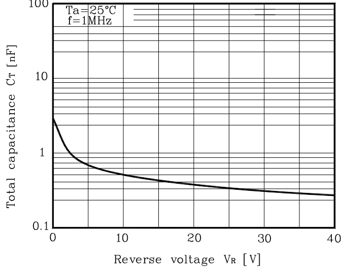
Fig. 4 C_T - V_R
