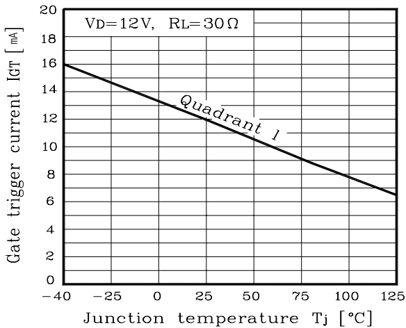
Fig. 5 I_{GT} - T_j
