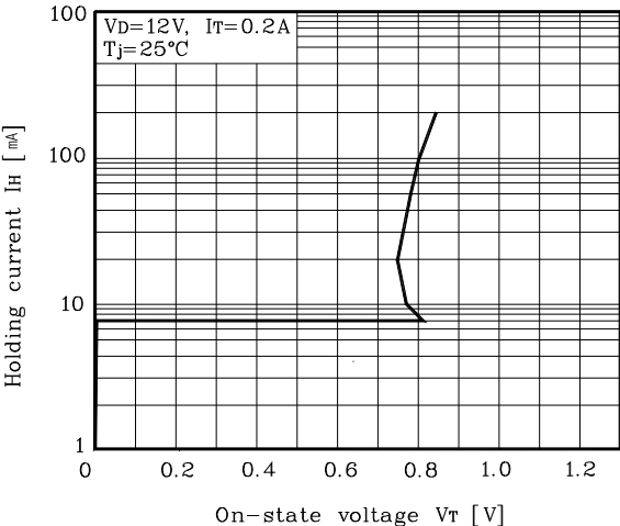
Fig. 9 I_H - V_T
