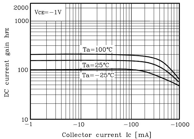
Fig. 4 h_{FE} - I_C
