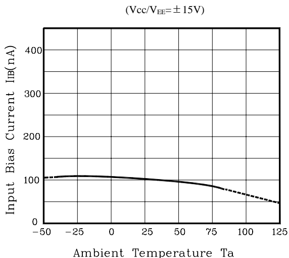
Fig. 3 I_B - T_a
