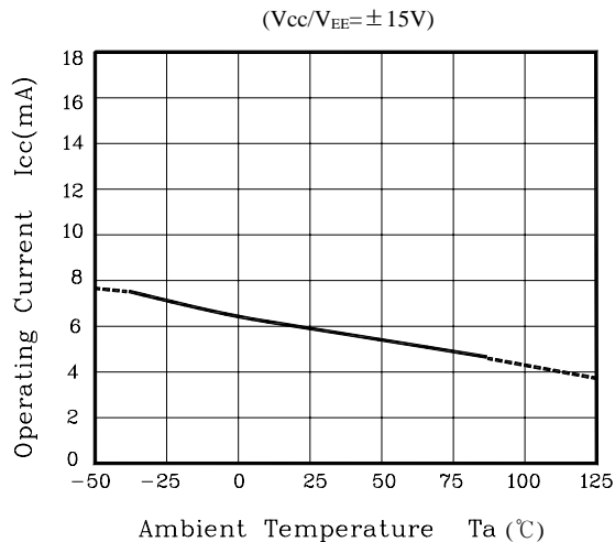
Fig. 8 I_{CC} - T_a
