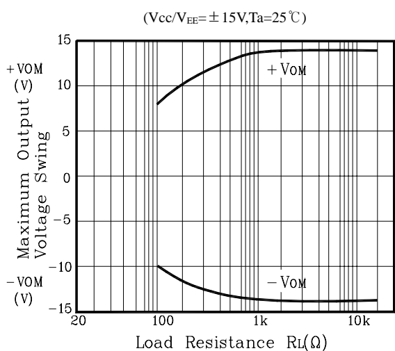
Fig. 5 V_{OM} - R_L
