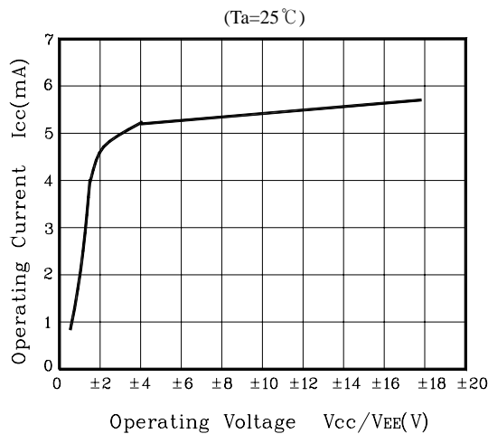
Fig. 10 I_{CC} - V_{CC}
