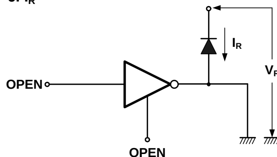
6. I_R
