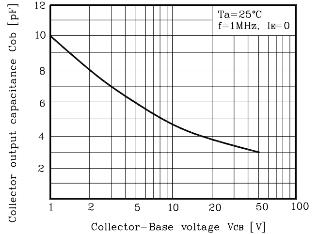
Fig. 4 C_{ob} - V_{CB}
