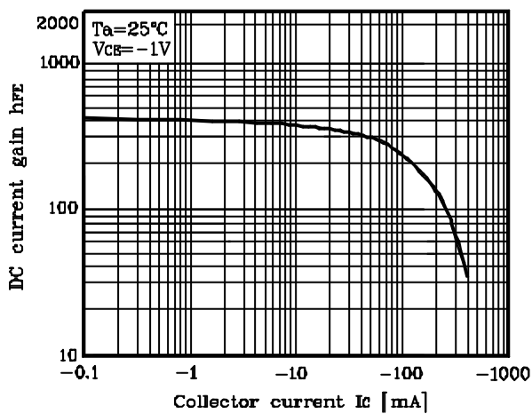
Fig. 3 h_{FE} - I_C
