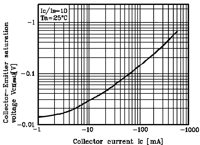
Fig. 5 V_{CE(sat)} - I_C
