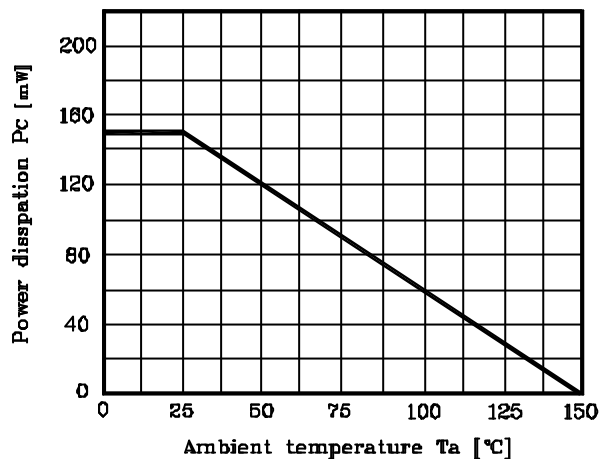
Fig. 1 P_C - T_a
