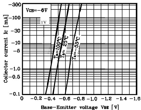
Fig. 2 I_C - V_{BE}
