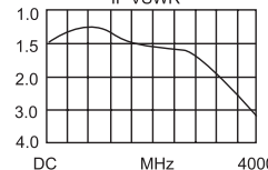
IF VSWR
