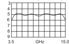
LO VSWR
