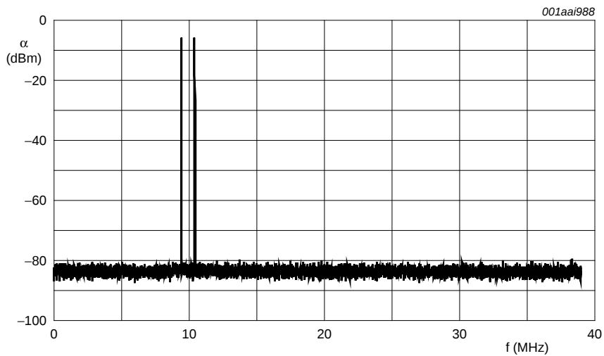
Fig 5. 2-tone SFDR
