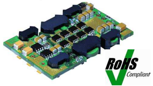
Q48S30018 Converter
