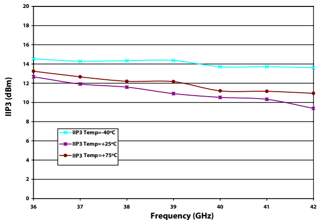
USB IIP3 for XU1006-QB Vg2=-0.5V, Vd=4V, Id=240mA, P_LO=+4dBm, P_IF/10MHz=-5dBm, ?F=10 MHz
