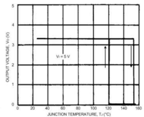
■ Thermal Protection
