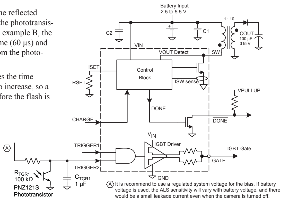
Figure 9. ALS typical application
