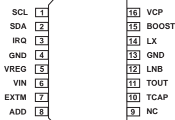
A8285SIB SOIC
