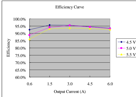
Vo=3.3 V
