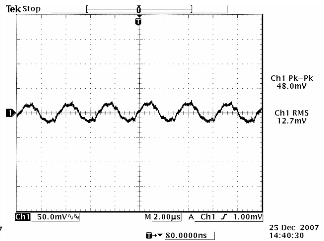
48 Vdc input
