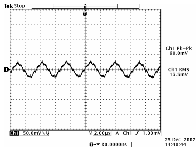
75 Vdc input
