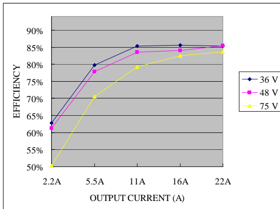
Vo=1.5 V
