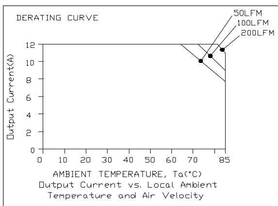
xRSB-40U02x, Vin=48V
