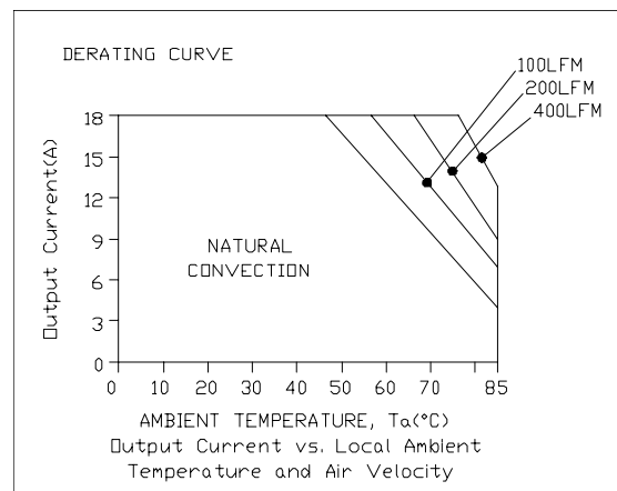
xRSB-40UV2x, Vin=24V
