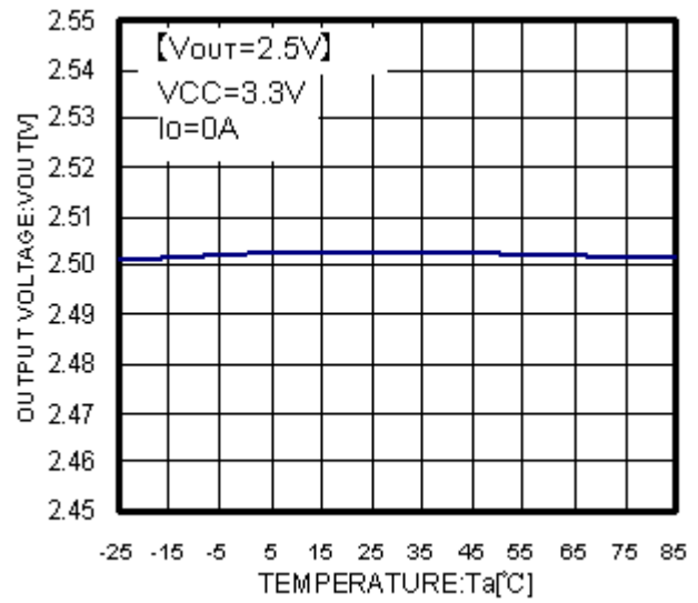
Fig.7 T a -V OUT
