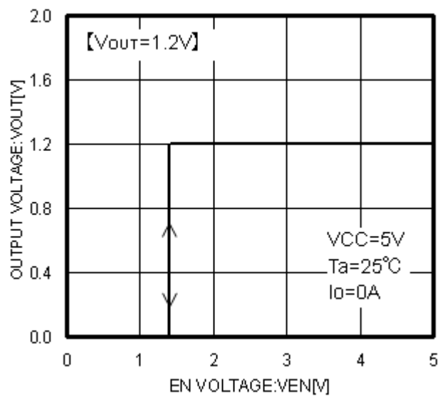
Fig.5 VEN - VOUT
