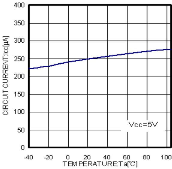
Fig.12 Ta-Icc
