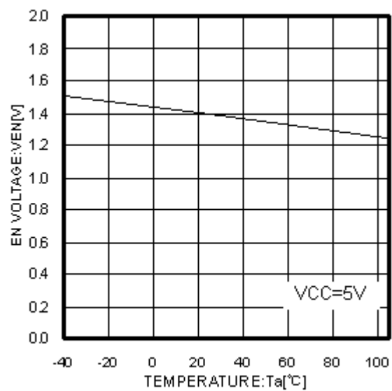
Fig.11 Ta - VEN
