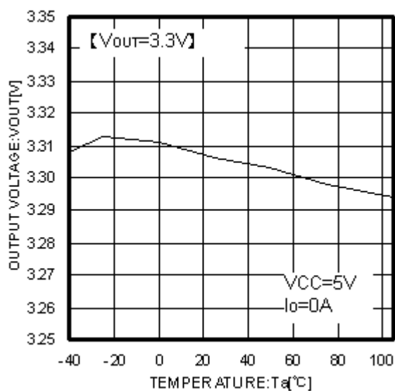
Fig.7 Ta - VOUT
