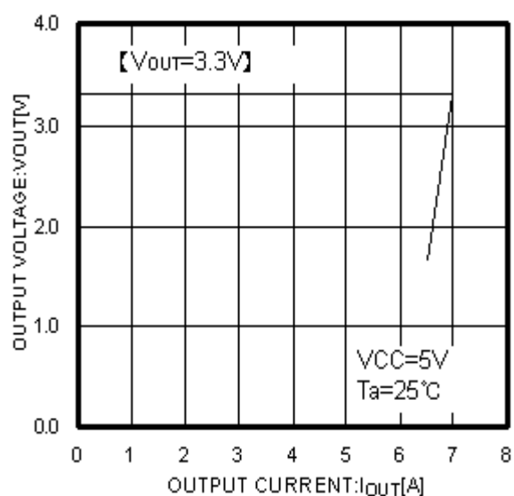
Fig.6 IOUT - VOUT
