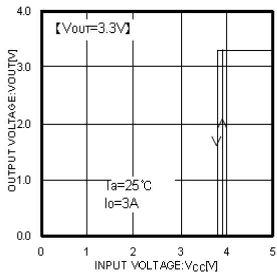
Fig.4 Vcc - VOUT
