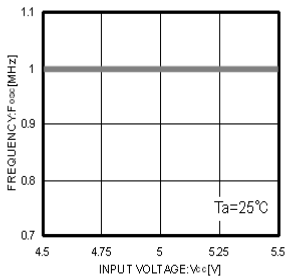
Fig.13 V_{cc} - F_{osc}
