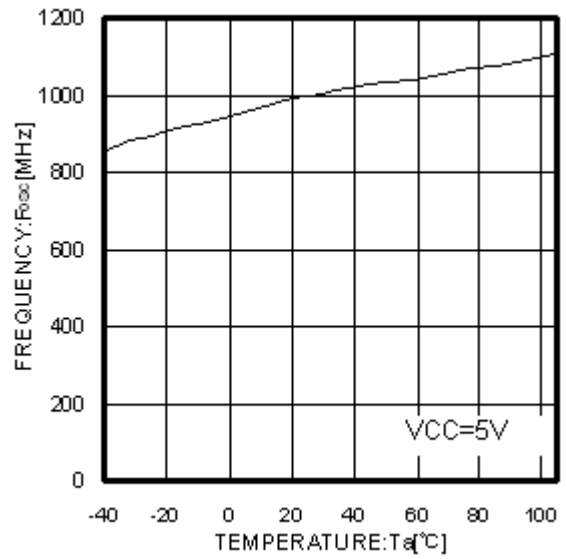
Fig.9 Ta - Fosc
