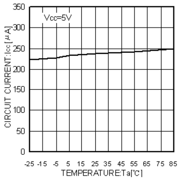
Fig.12 T_a - I_{cc}
