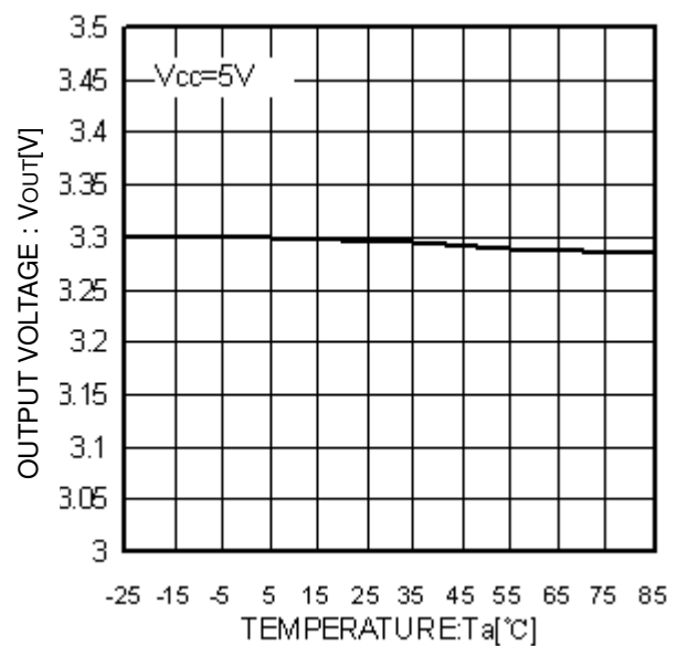
Fig.7 Ta-Vout
