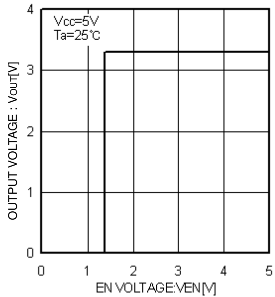
Fig.5 Ven-Vout
