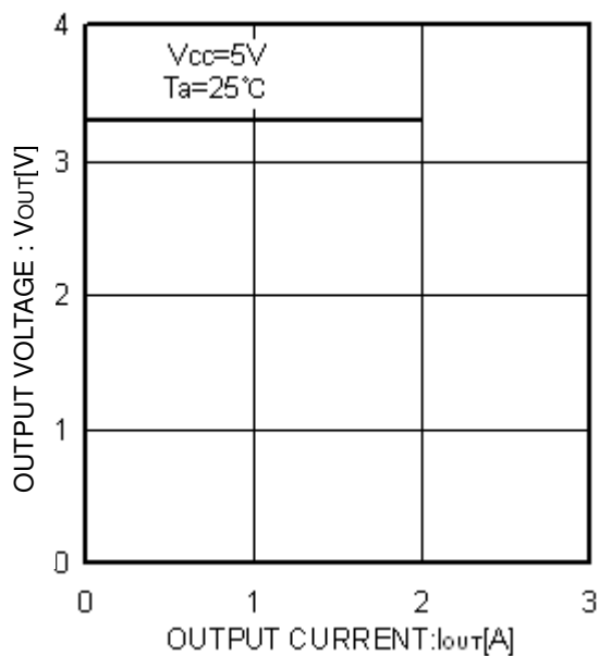
Fig.6 Iout-Vout
